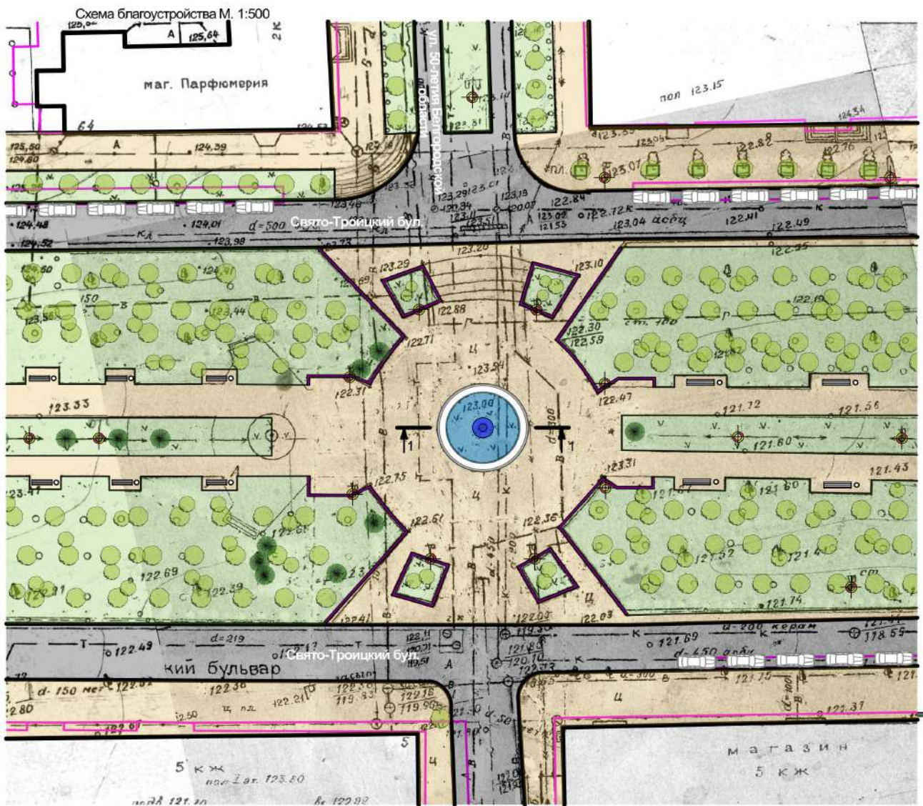
Ситуационная схема
